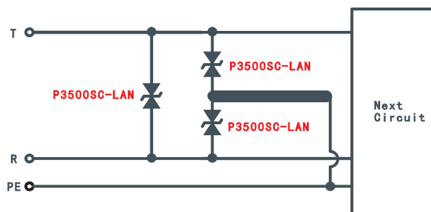
POS机防护方案
