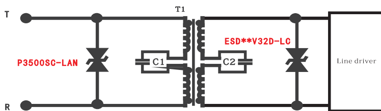
VDSL防护方案
