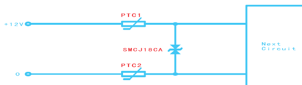
DC12V电源防护方案
