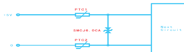
DC5V电源防护方案
