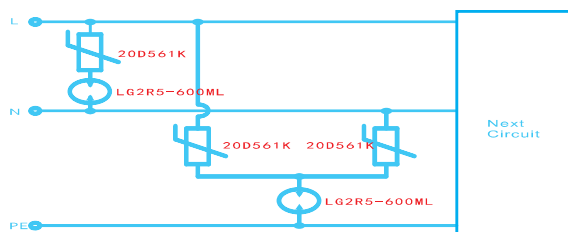
AC220V电源防护方案
